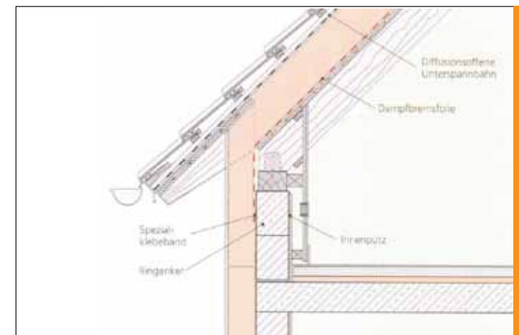
9 Kniestock mit Installationsebene (Luftundichtigkeit von Wohngebäuden, RWE Energie, Essen 1996)
