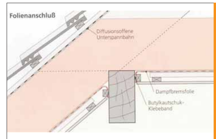
8 Anschluss der luftdichten Ebene an eine freiliegende Mittelpfette (Luftundichtigkeit von Wohngebäuden, RWE Energie, Essen 1996)
