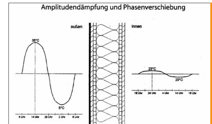
12 Effektivität bei Amplitudendämpfung und Phasenverschiebung
