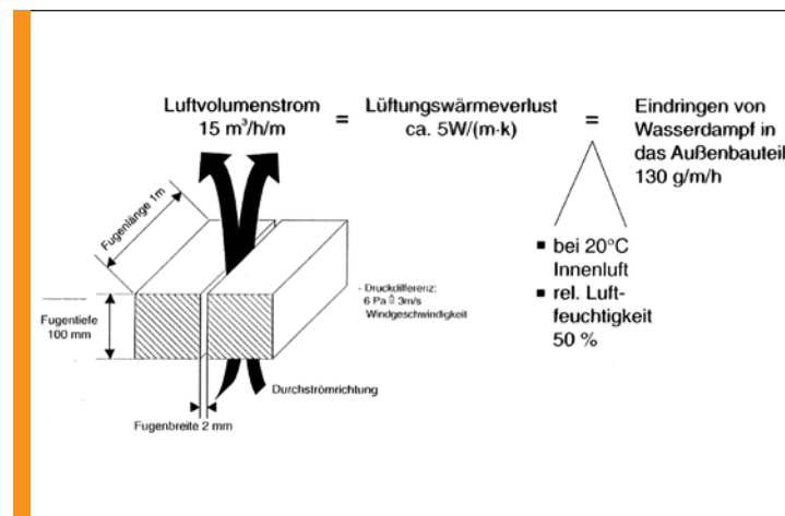
7 Wirkung von Luftundichtheit in einer Fuge
